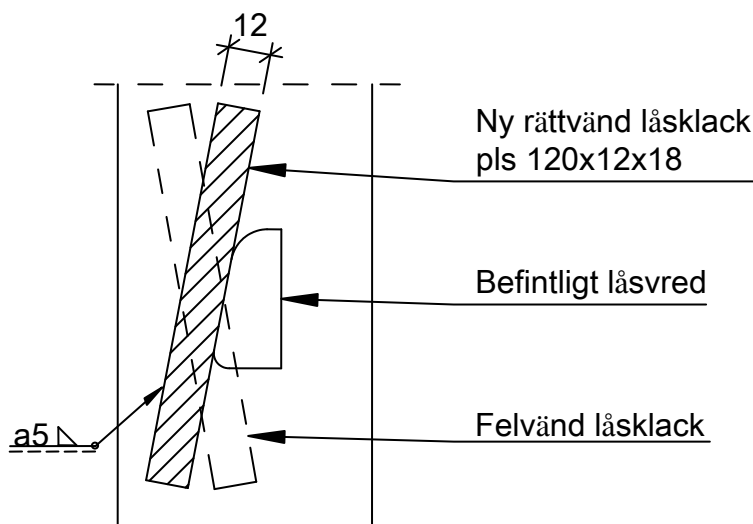
Figur T04-401a. Vertikalsnitt genom låsklack.
