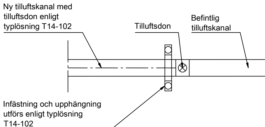
Figur T14-104a. Förlängning av befintlig tilluftskanal.
